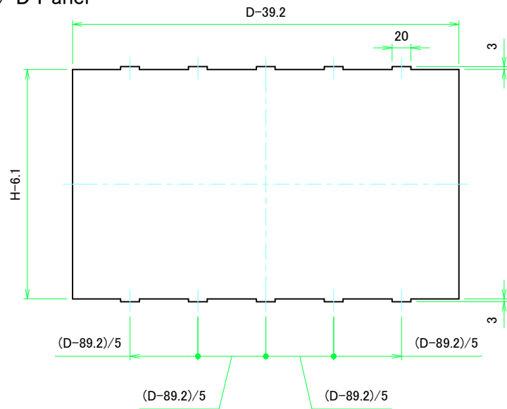
Dパネル1表面 / D Panel 1 Frontside
